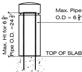
PERIMETER SECURITY (D) ANTI - RAM
